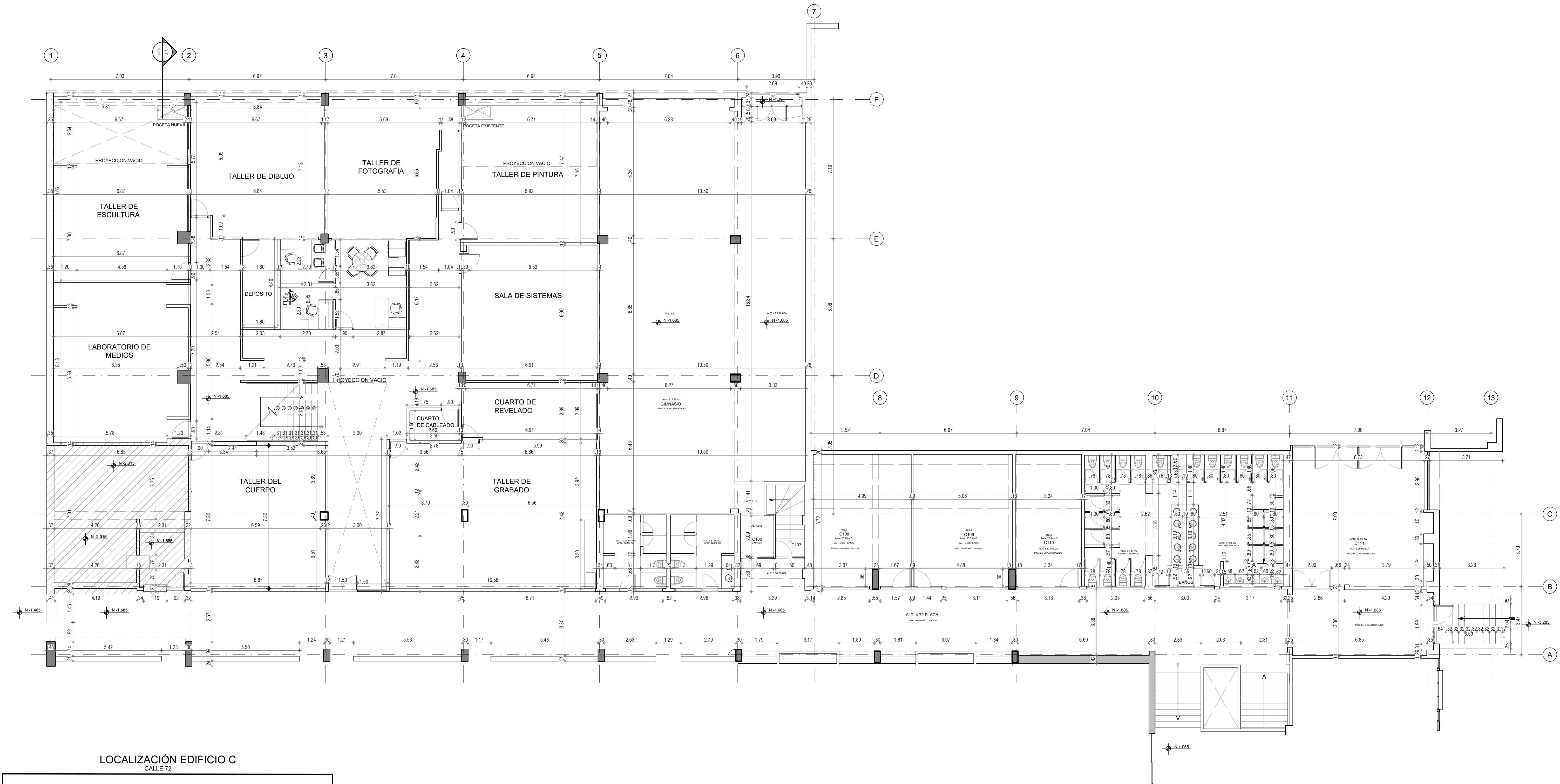
EDIFICIO-C PRIMER PISO ESC _____ 1:100
