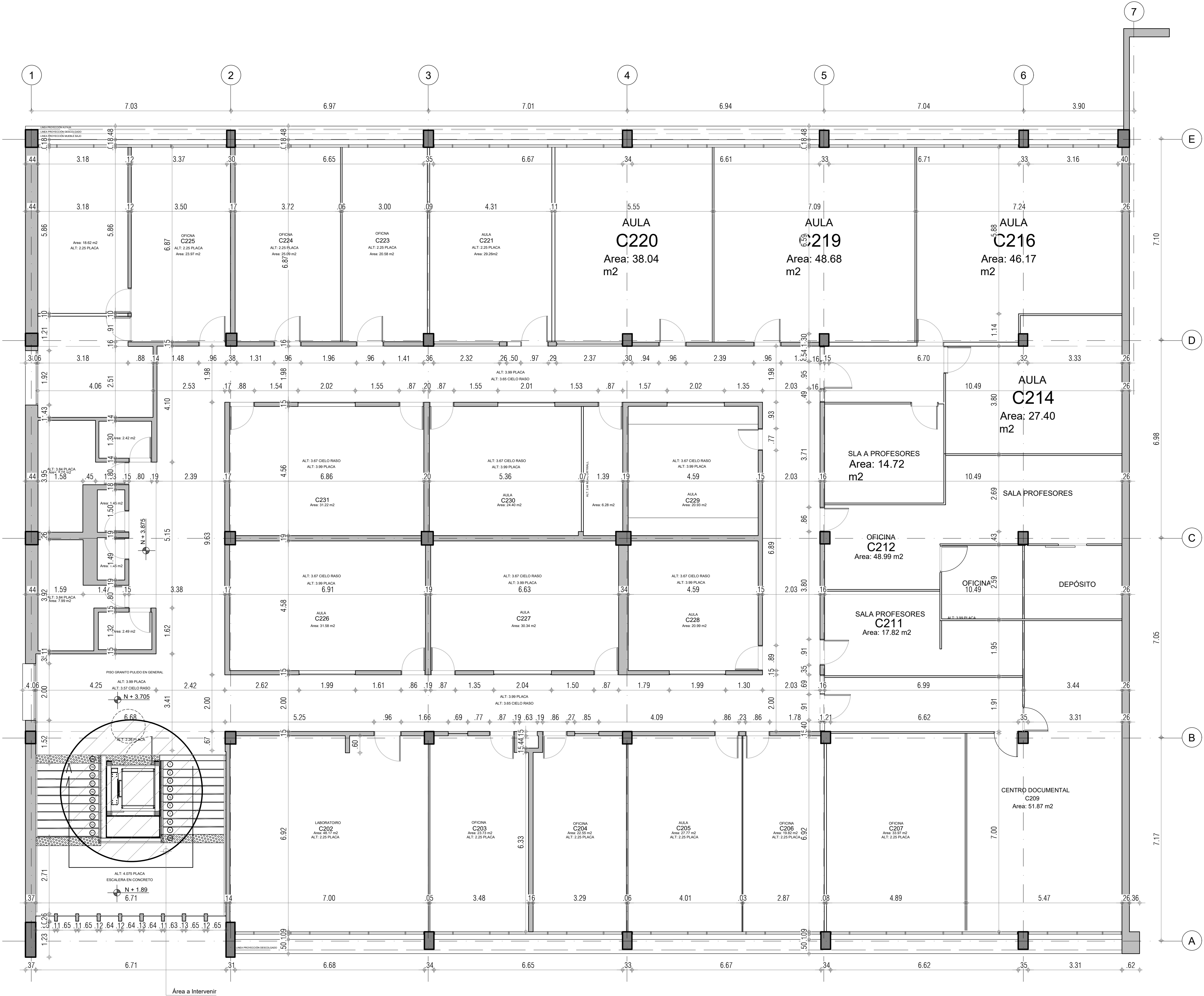
EDIFICIO-C EDU. SEGUNDO PISO ESC 1:75
