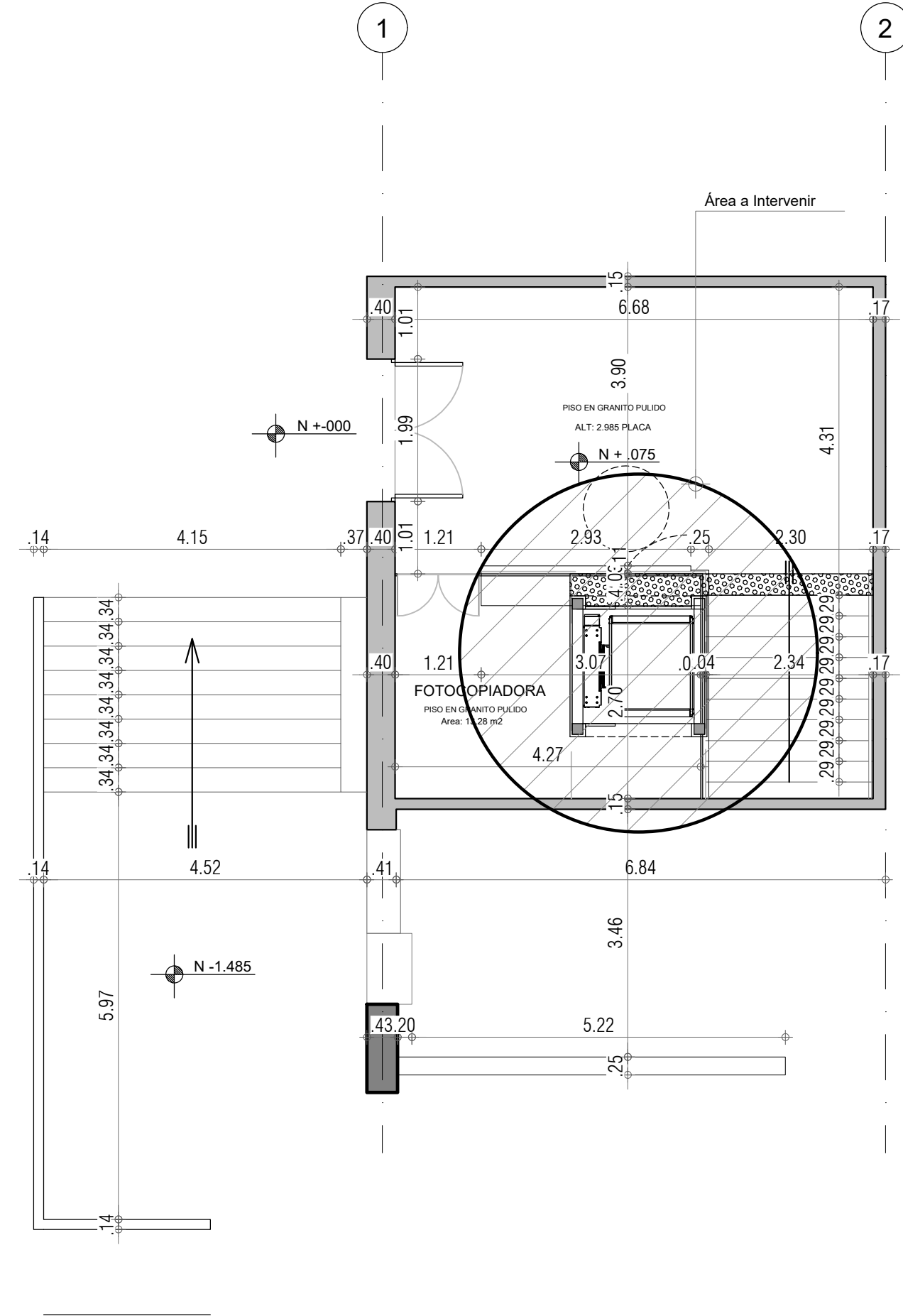
A-101 EDIFICIO-C EDU. PRIMER PISO ESC 1:75
