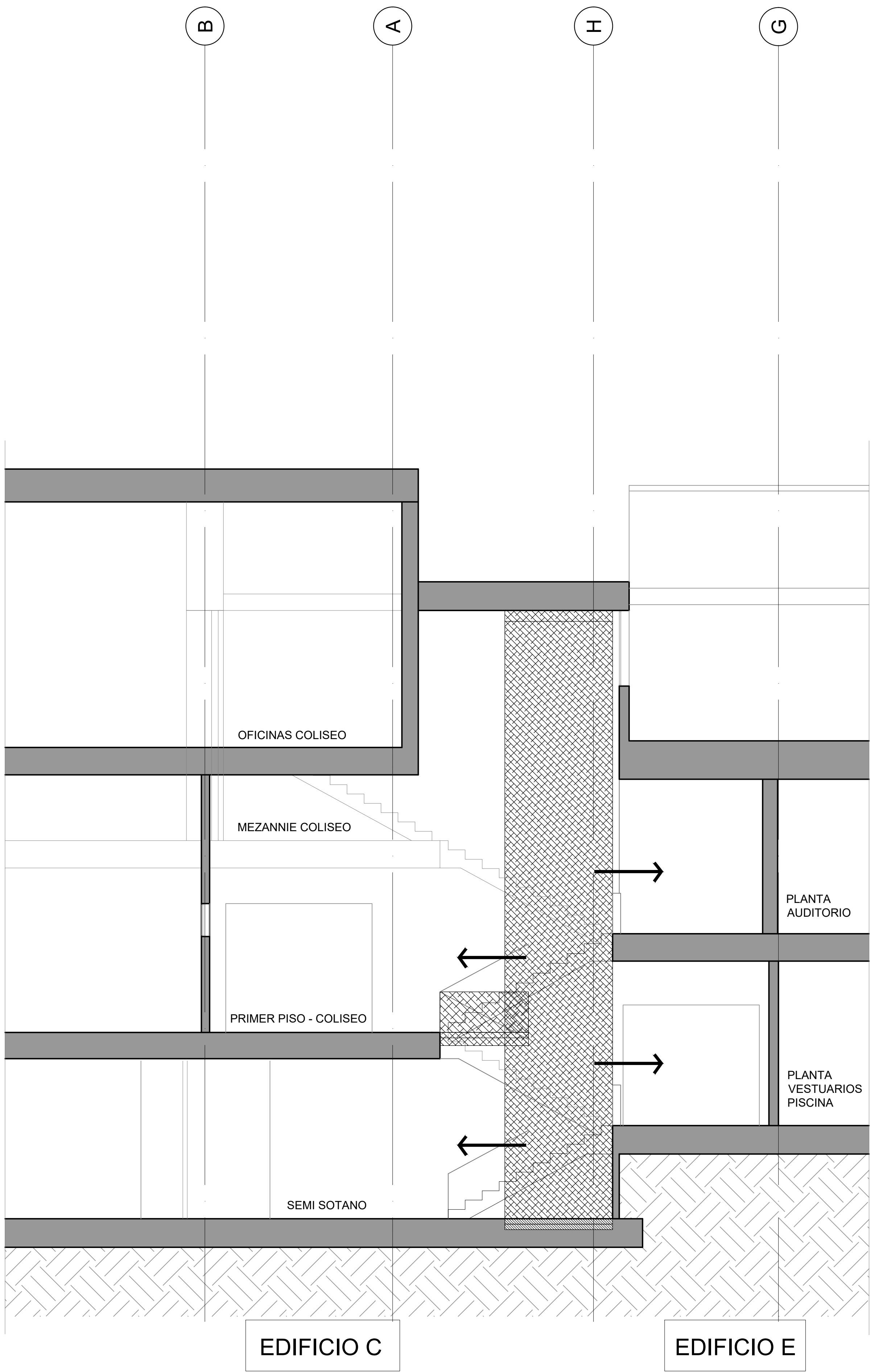
CORTE PROPUESTO HUECO ESCALERAS EDIFICIO C - E ESC _____ 1:50
