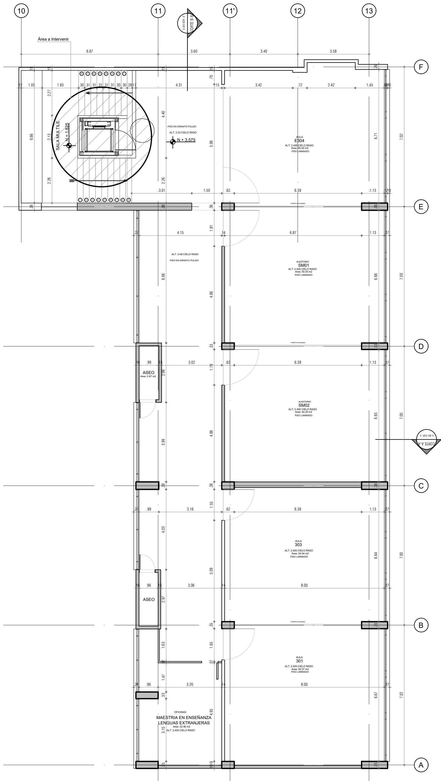
EDIFICIO-E TERCER PISO ESC 1:100
