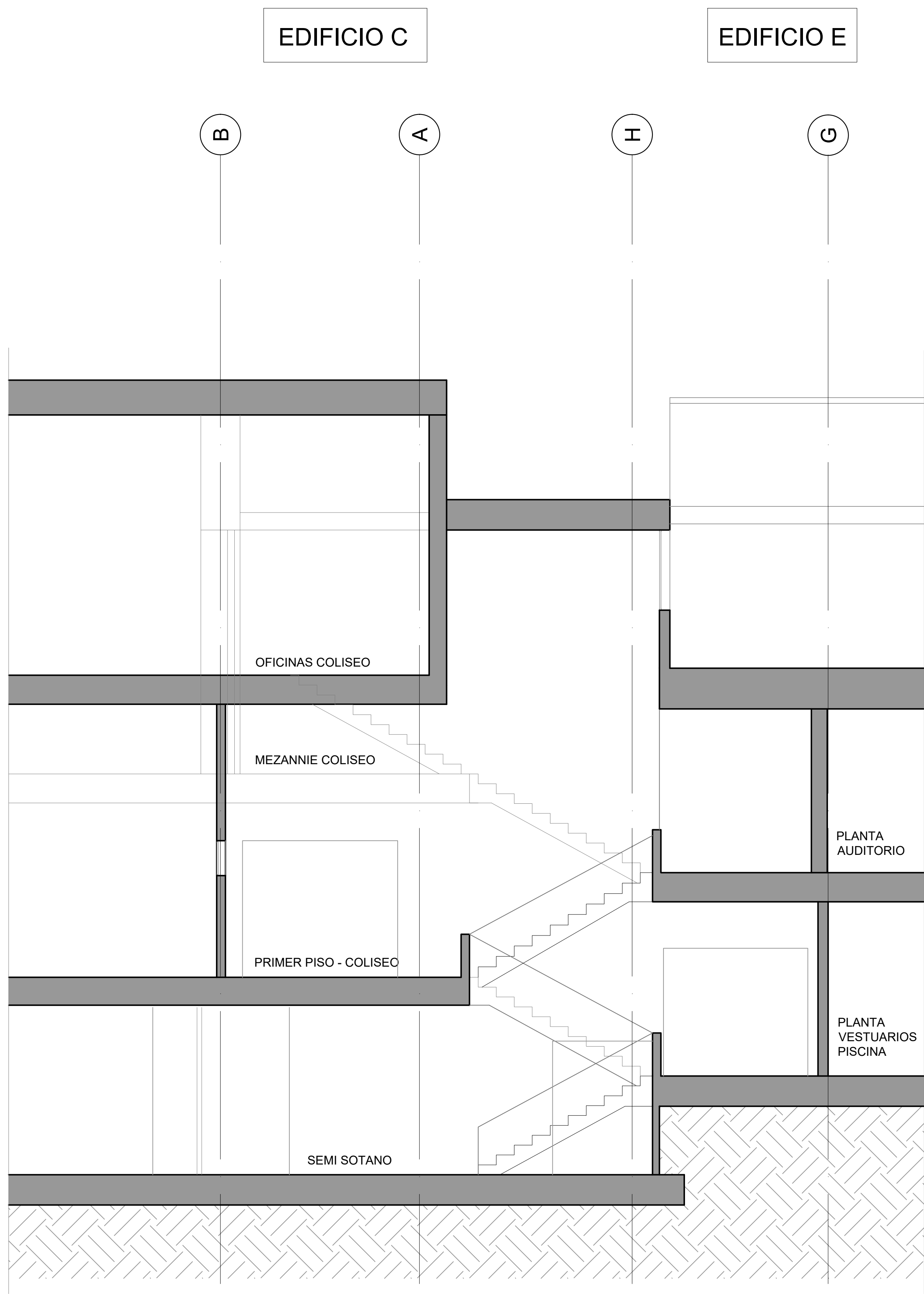
CORTE ACTUAL HUECO ESCALERAS EDIFICIO C - E ESC _____ 1:50
