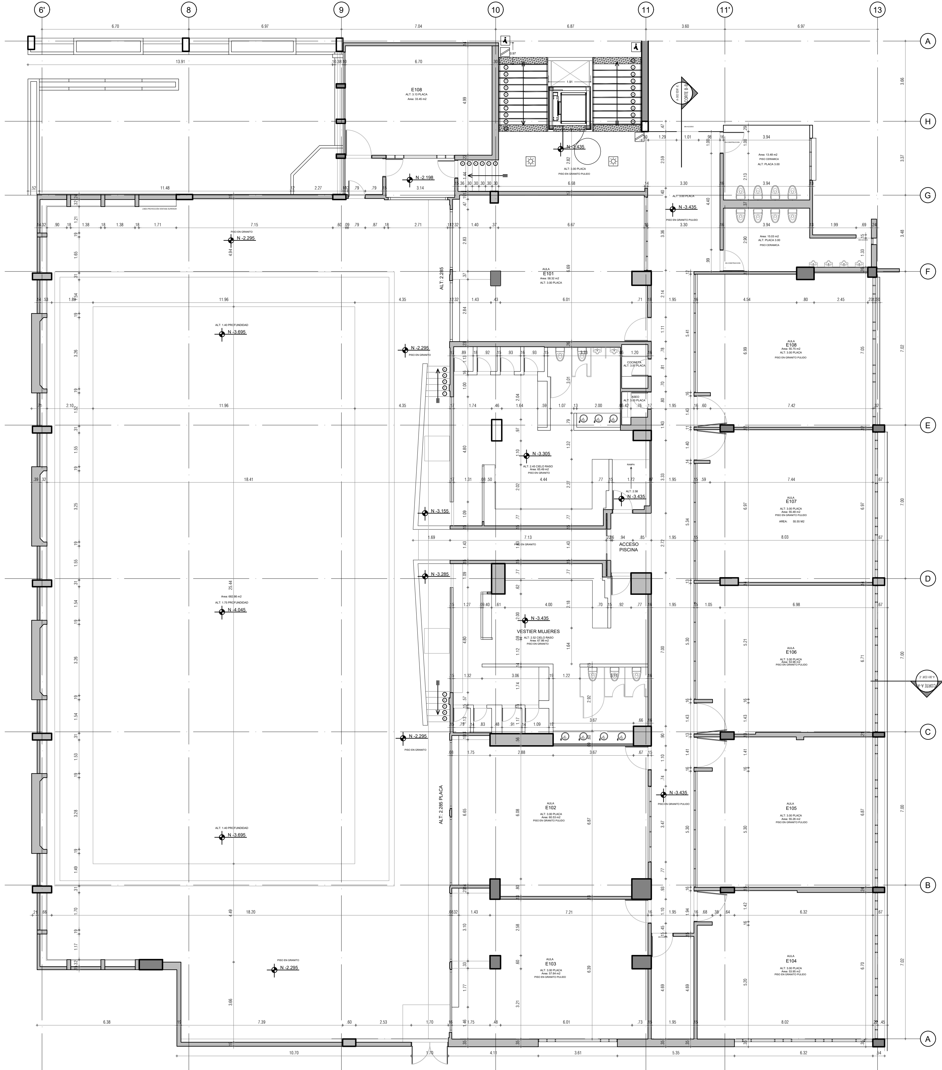
EDIFICIO-E PRIMER PISO ESC 1:100
